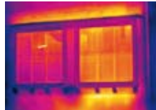
Gebouwen: warmteverlies
